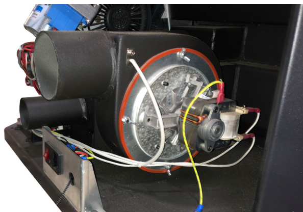
Figure 27 Ventilateur d'échappement du modèle PSBF66W
