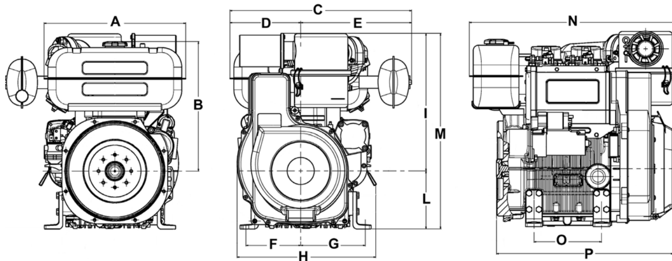
Dimension mm (in.) - DIMENSIONI MM - MESURES MM - EINBAUMASSE MM - DIMENSIONE MM - DIMENÇÕES (MM)
