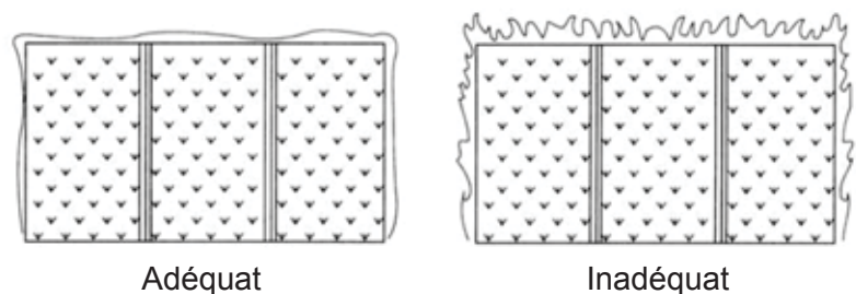
FIGURE 5 Flamme appropriée du brûleur
