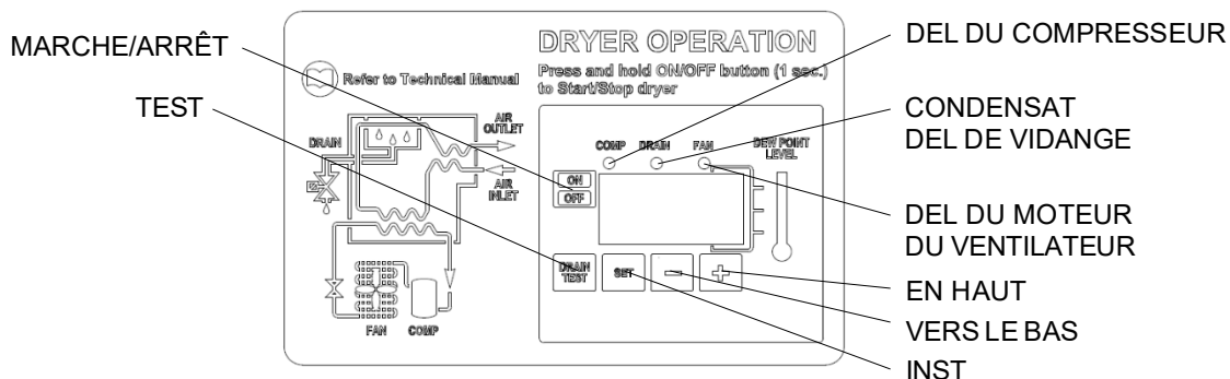
PHOTO 1 VISUALISATION DE L’AFFICHAGE ET VOYANTS DEL DE SIGNALISATION
