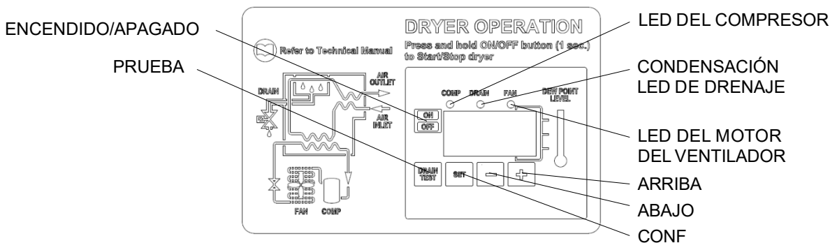
IMAGEN 1 PANTALLA LED DE VISUALIZACIÓN Y SEÑALIZACIÓN
