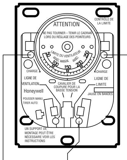
INTERRUPTEUR-LIMITEUR Honeywell
