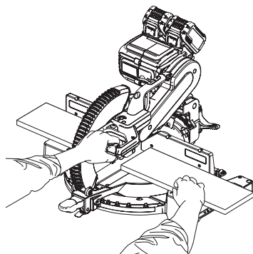
CORTE CORRECTO
