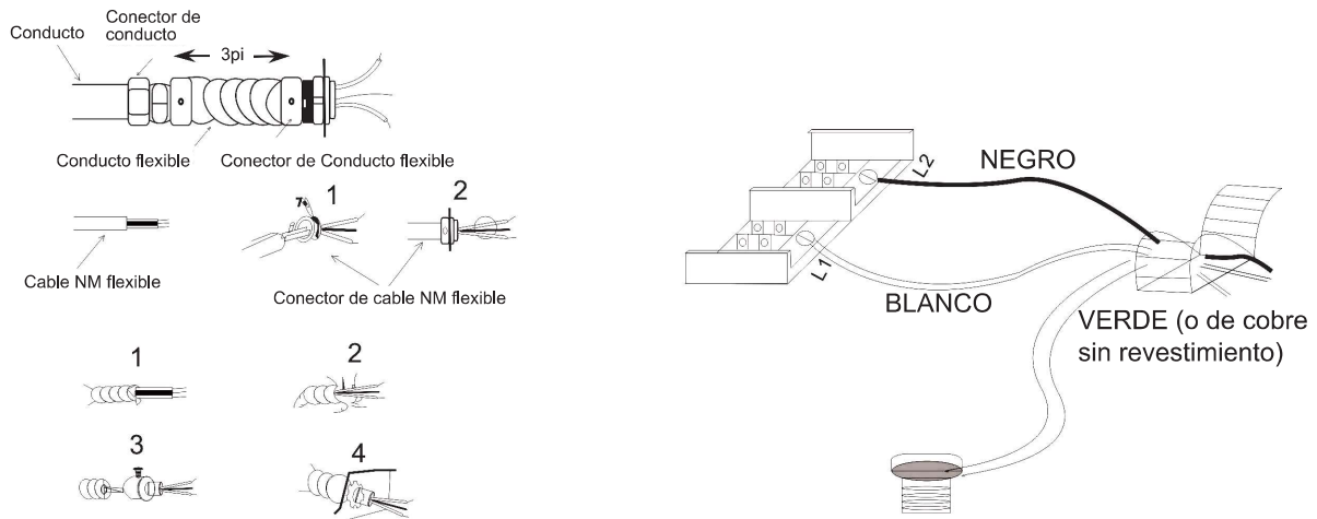
Conectores, cable y demás elementos utilizados para el cableado del calefactor
