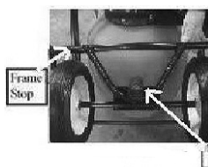
Figure 3. Rotate Pivot Mount Plate onto Frame Stop Figura 3. Gire la placa de montura del pivote hacia la parada del chasis.
