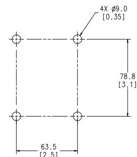
Posición de los pernos de montaje
