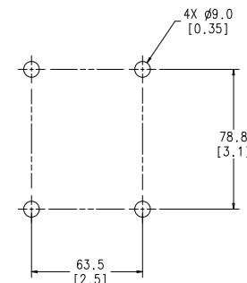
Entraxes de fixation
