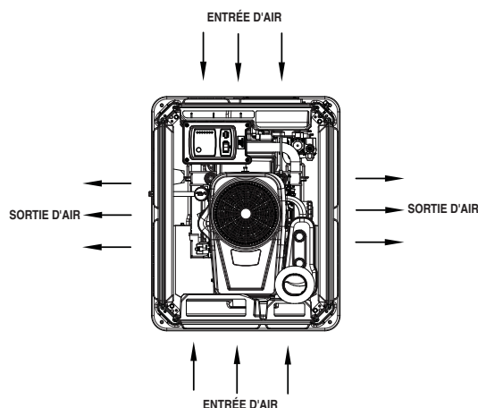
Schéma 4.4 - Emplacements des événements de refroidissement
