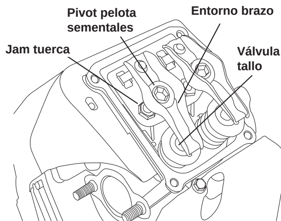
Figura 4.9 - Ajuste de la holgura de la válvula
