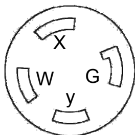
Figure 3. Prise à verrouillage par rotation NEMA L14-30R : 240/120 volts, 30 A
