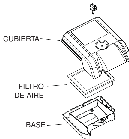
Figura 24 - Filtro de aire de 10kW (Nº de parte 073111)
