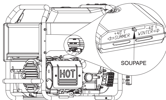
Figure 9 - Soupape d'été/hiver
