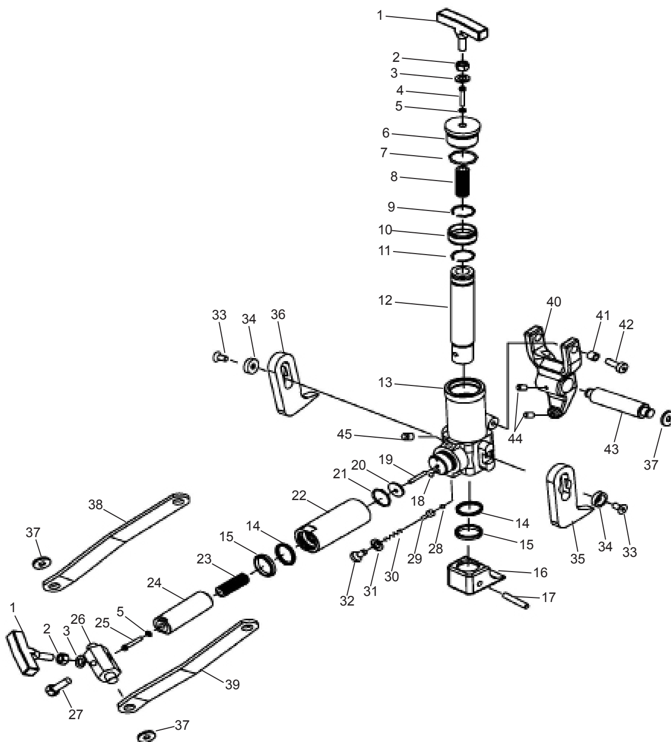
Figure 4 : Illustration des pièces de rechange du modèle 22910
