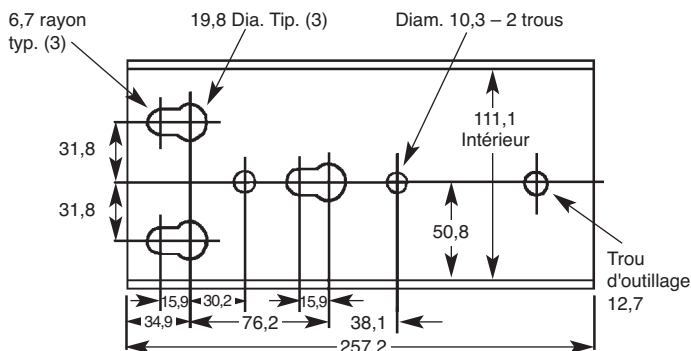
FIGURE 3 Schéma des trous du socle (mm) Modèles SA9000AC et SA12000AC
