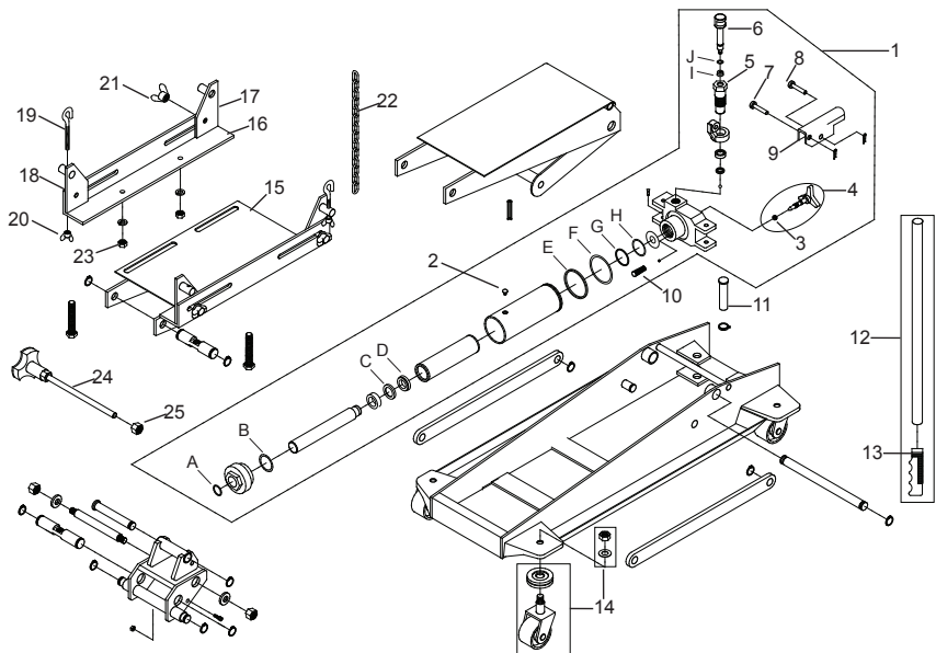
Figura 4: Ilustración de piezas de repuesto para el modelo 41100C
