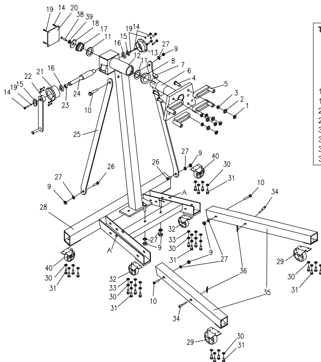
Figura 6: ilustración de ensamblaje para el modelo 31256
