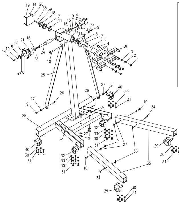
Figure 6 : Illustration d'assemblage du modèle 31256
