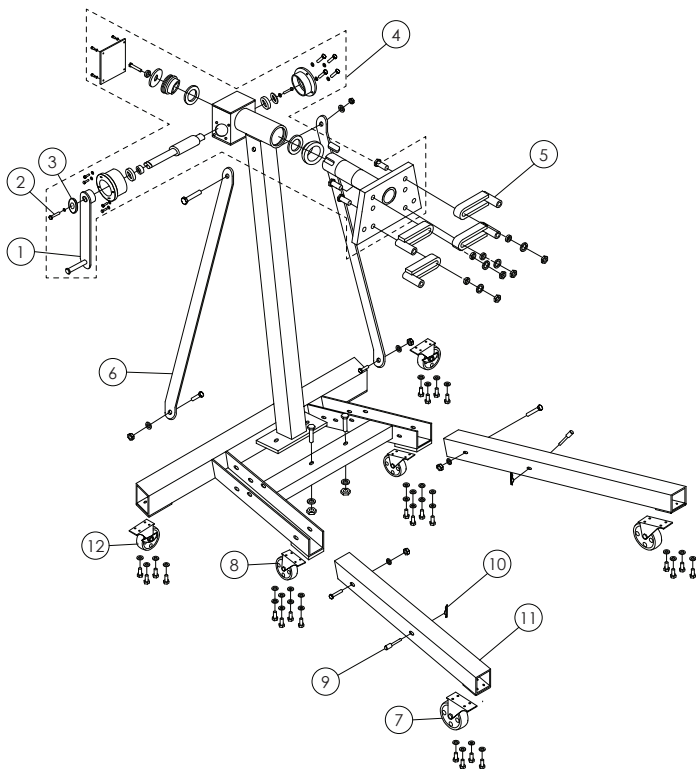
Figure 10 : Illustration des pièces de rechange du modèle 31256
