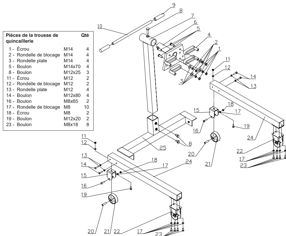
Figure 5 : Illustration d'assemblage du modèle 31250
