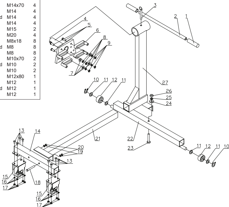
Figura 4: ilustración de ensamblaje para el modelo 30750
