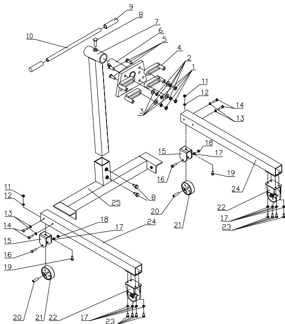
Figure 9 : Illustration des pièces de rechange du modèle 31250
