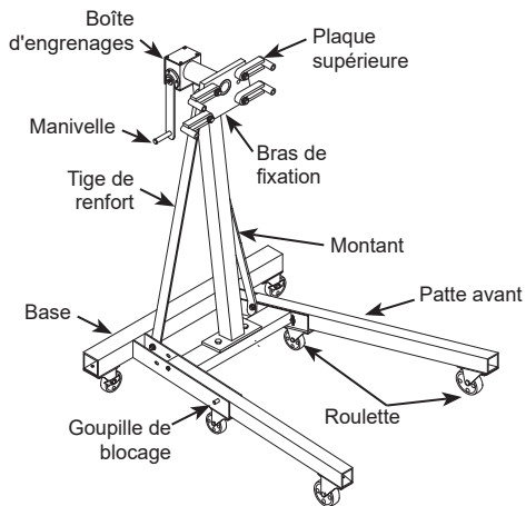
Figure 3 : Composants du modèle 31256
