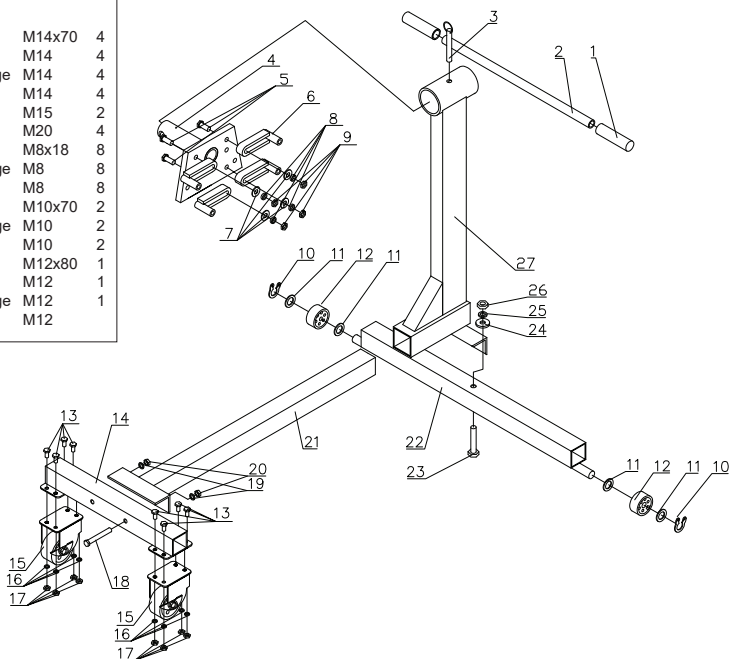
Figure 4 : Illustration d'assemblage du modèle 30750
