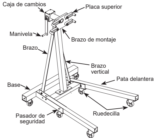
Figura 3: componentes del modelo 31256
