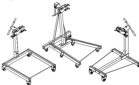
Figure 7 - Limites périphériques de charge des supports
