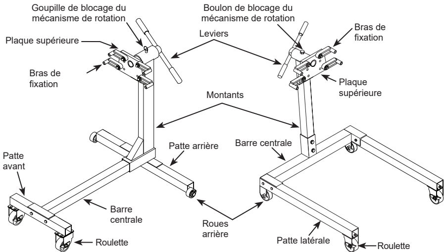
Figure 1 : Composants du modèle 30750
