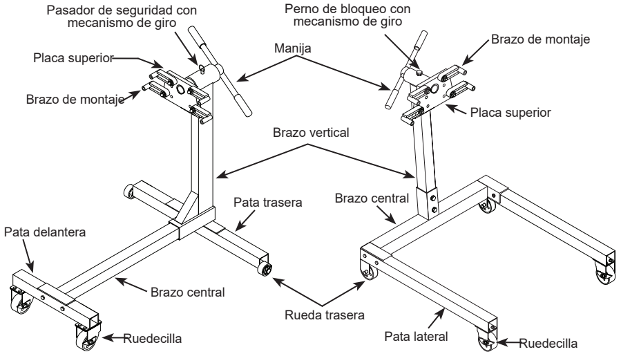
Figura 1: componentes del modelo 30750
