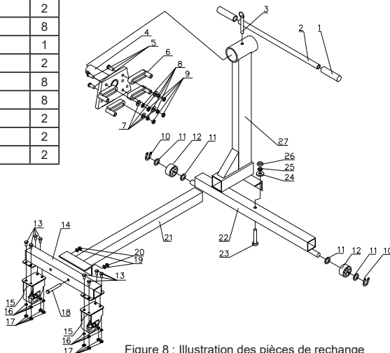
Figure 8 : Illustration des pièces de rechange du modèle 30750
