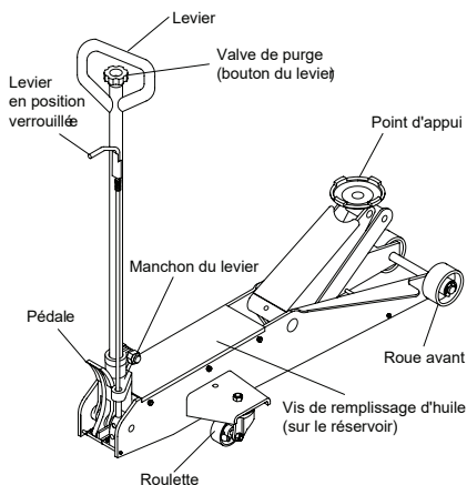
Figure 1: Composants des modèles 25057 et 25107
