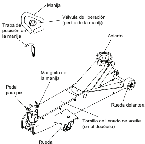
Figura 2: Componentes de los modelos 25057 y 25107
