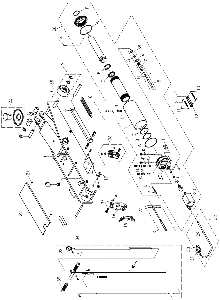
Figure 3 : Illustration des pièces de rechange des modèles 22100C et 22101C
