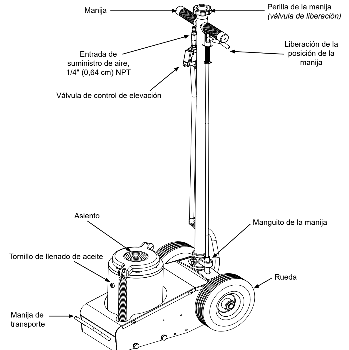
Figura 1: Nomenclatura habitual de un gato para camiones (se muestra 23227)
