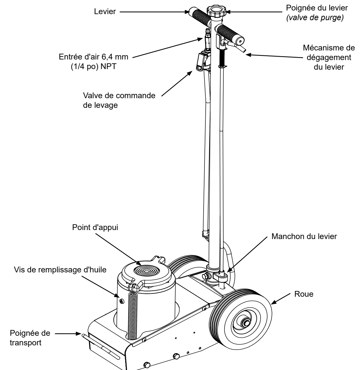
Figure 1 : Pièces d'un cric hydraulique standard pour camion (modèle 23227 illustré)
