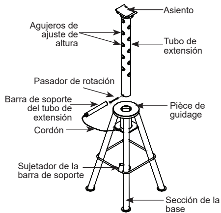
Figure 1 : Componentes de los modelos 32105B y 32107B
