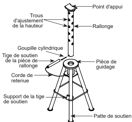
Figure 1 : Composants du Modèles 32105B et 32107B
