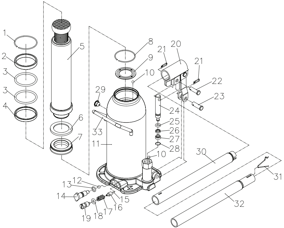
Piezas de repuesto para los modelos 10025W, 10045W, 10065W, 10125W, 10205W
