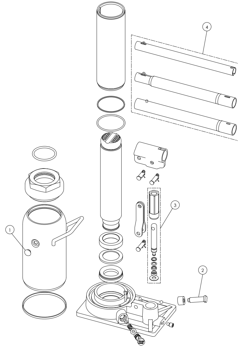
Figura 2: Ilustración de piezas de repuesto para los modelos 10120, 10128, 10200 y 10208
