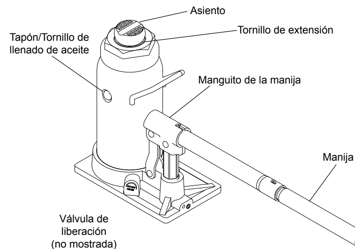
Figura 1: Nomenclatura habitual de un gato de botella en línea
