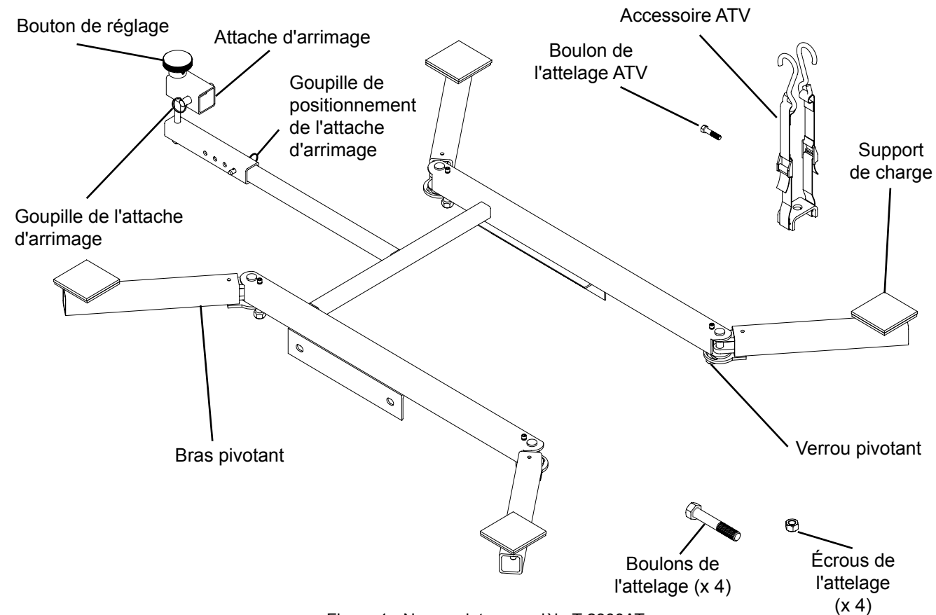
Figure 1 - Nomenclature modèle T-2300AT
