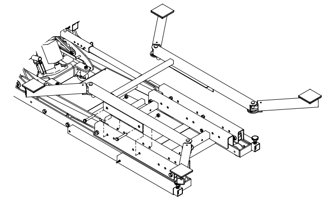
Figura 2: Montaje del accesorio para fijación UTV.
