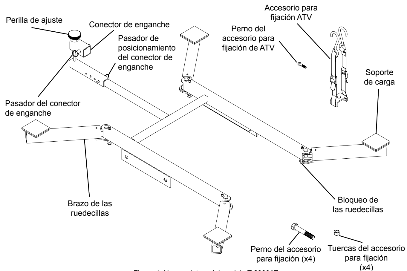
Figura 1: Nomenclatura del modelo T-2300AT
