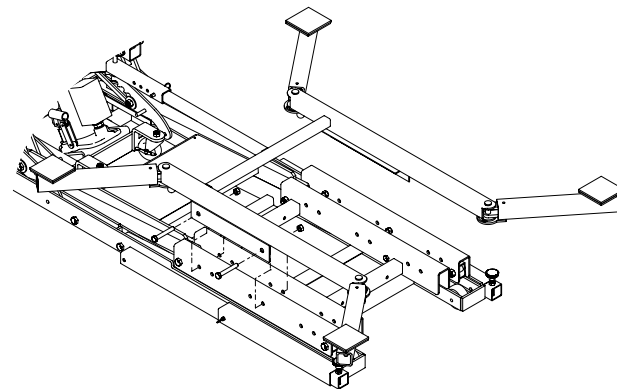
Figure 2 : Assemblage de l'accessoire UTV
