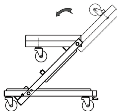
Figure 3 - Schéma de l'ajustement du sommier en siège
