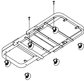
Figure 2 - Colocación de las Ruedecillas
