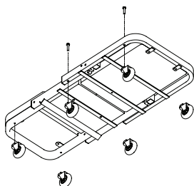
Figure 2 - Attacher les roulettes du sommier
