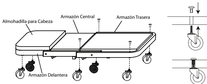
Figure 1 - Modelo B2036 Partes
