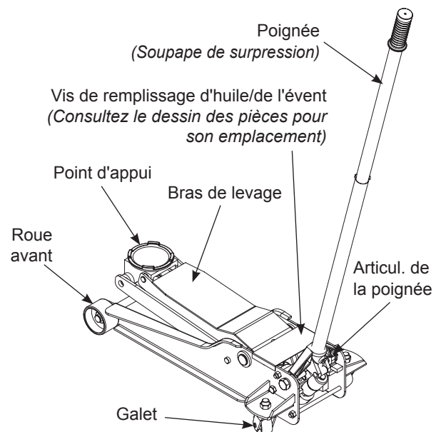
Figure 1 : Pièces d'un cric typique
