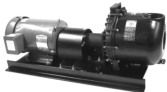
Impulsor eléctrico y acoplamiento largo
